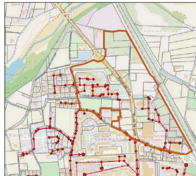
Réseau d'eaux usées
