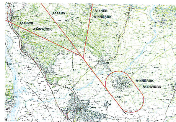
Trajectoires d'approche au QFU 14 (face au sud-est), avec : ▪ des approches de type « break » effectuées à 1 500 pieds par les avions de chasse (A14NERBK, A14NWRBK), ▪ une approche aux instruments « IFR » (A14AMV), ▪ des approches à vue (A14NWR, A14NER).
