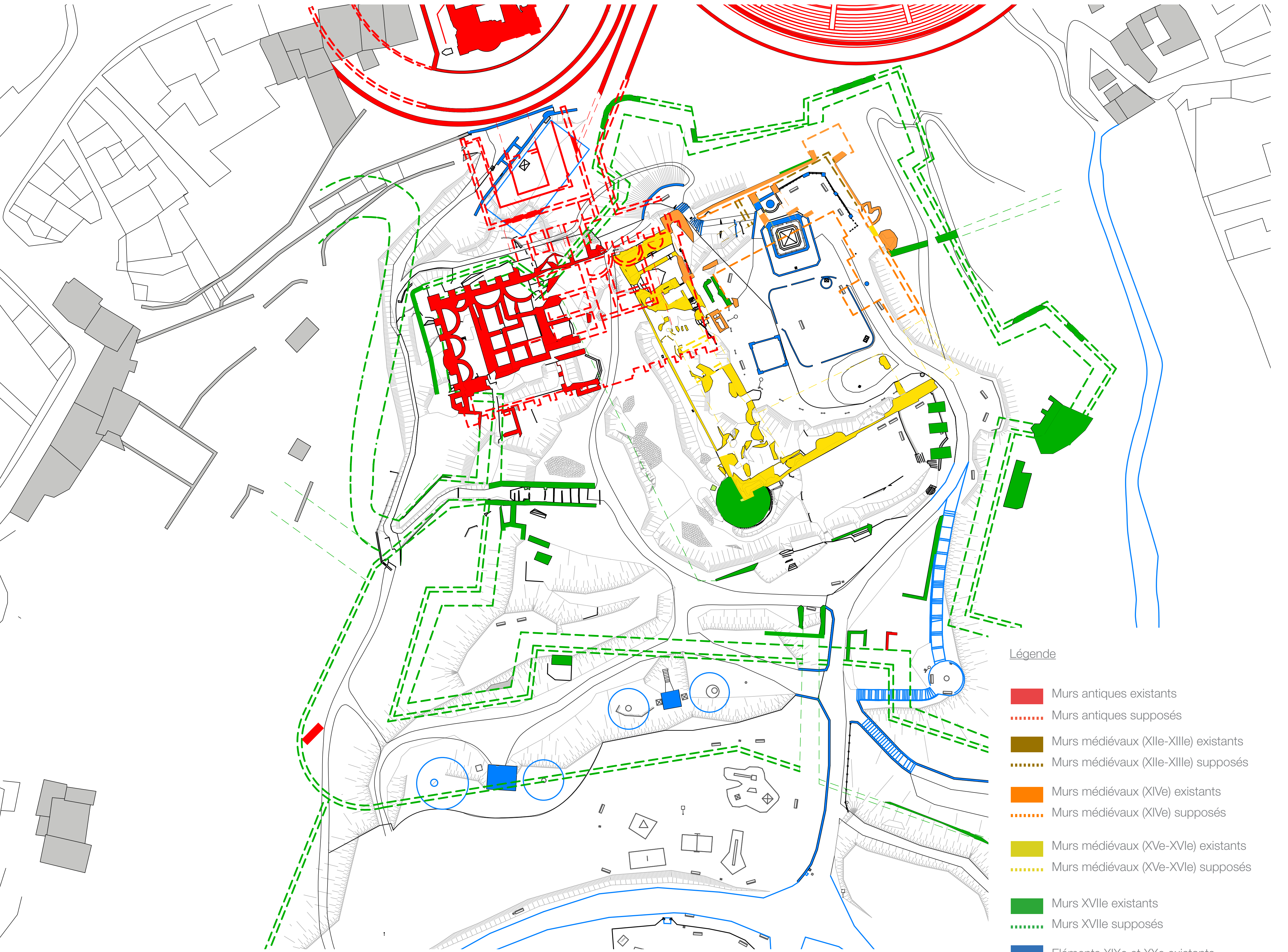
Hypothèse de restitution à partir des plans d'archives connus, échelle 1:500
